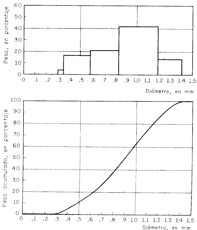
Fig 2. Distribución de densidad y distribución acumulada de la alúmina activada empleada en el ensayo 3
