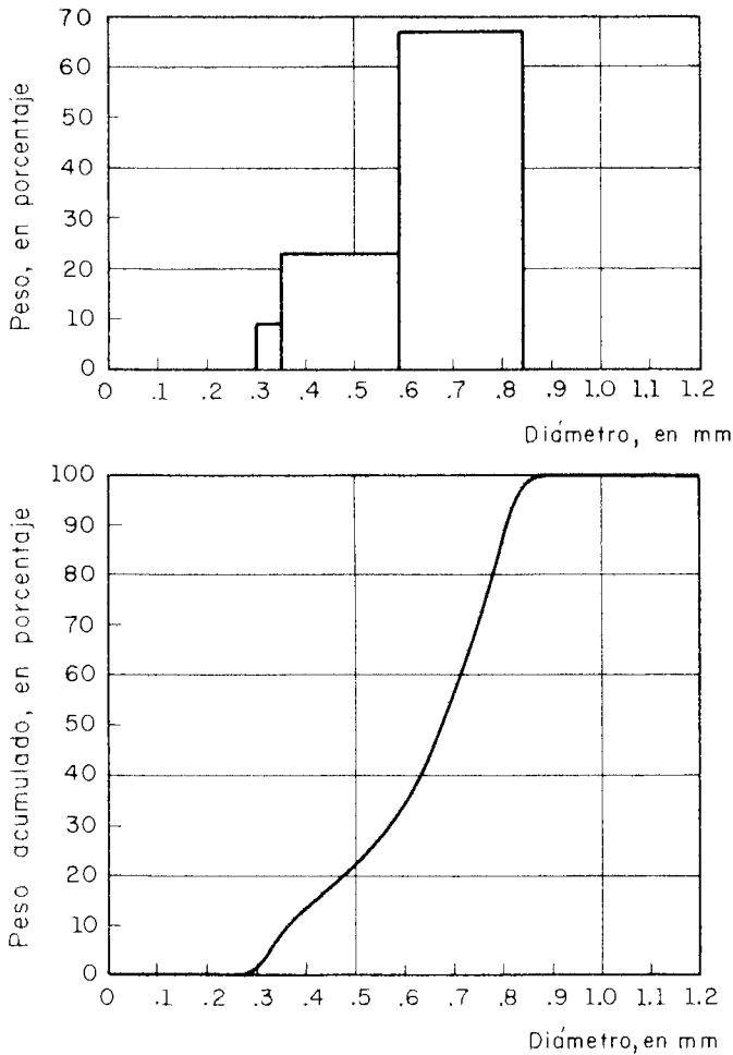
Fig 3. Distribución de densidad y distribución acumulada de la alúmina activada empleada en los ensayos 4 y 5
