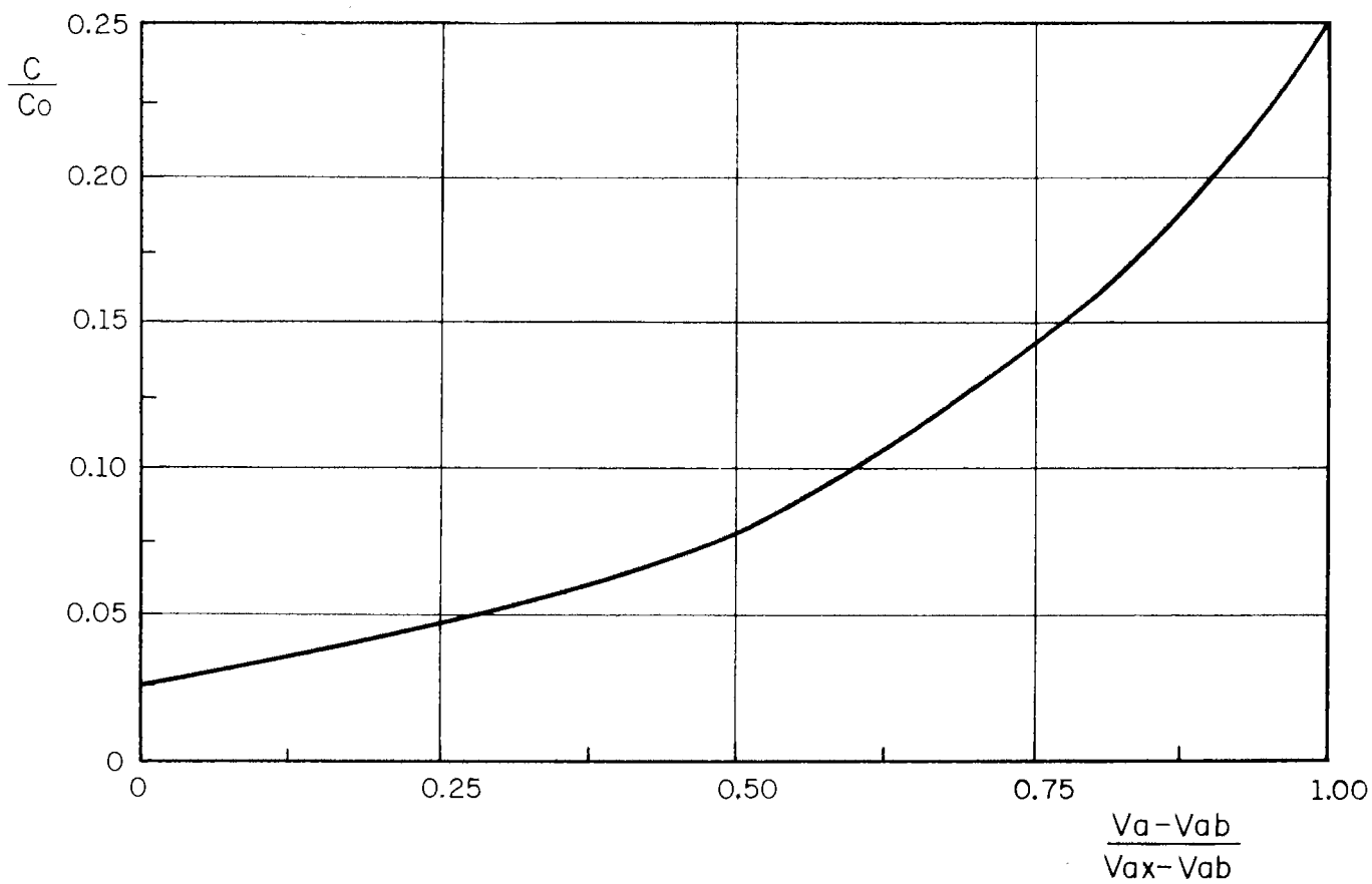
Fig 7. Adsorción de arsénico con alúmina activada. Ensayo 4. Curva de funcionamiento de la columna en la zona de adsorción
